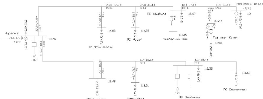
Рисунок 3.2.2.13 – Нормальный режим. Зимний максимум 2022 г.
