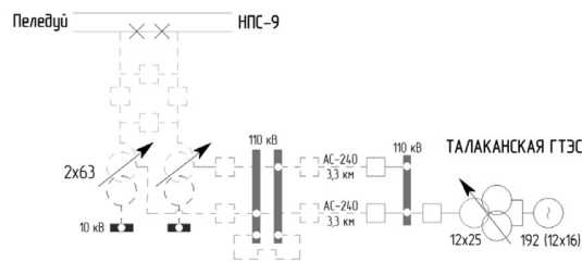
Рисунок 3.6.1 – Схема подключения Талаканской ГТЭС
