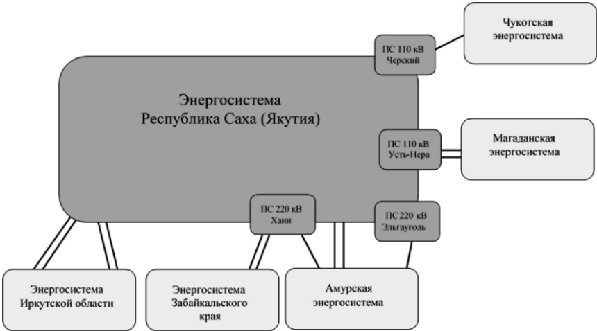
Рисунок 2.16.1 – Блок-схема внешних электрических связей Республики Саха (Якутия)
