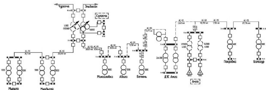
Рисунок 3.2.2.9 – Принципиальная схема электрических сетей 35 кВ и выше
