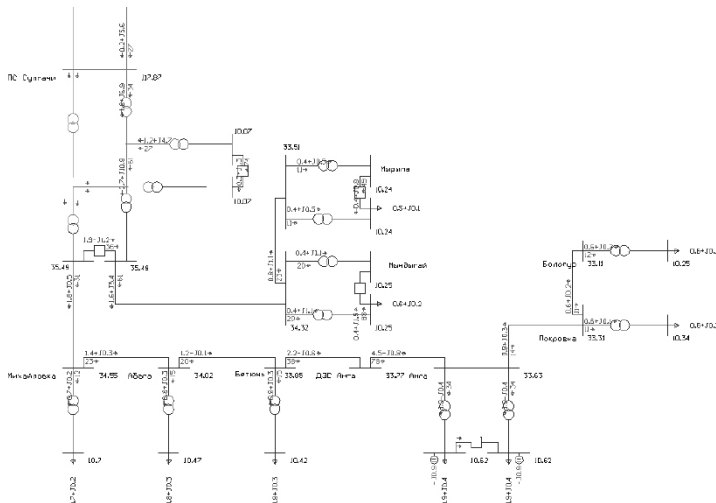
Рисунок 3.2.2.5 – Нормальный режим. Зимний максимум 2021 года
