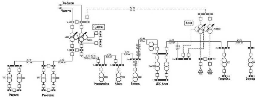
Рисунок 3.2.2.11 – Принципиальная схема электрических сетей 35 кВ и выше
