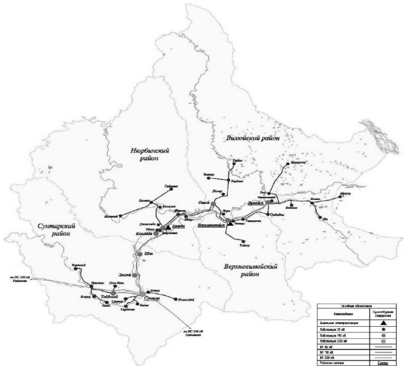
Рисунок 3.2.2.1 – Карта-схема электрических сетей 35 кВ и выше рассматриваемого энергорайона
