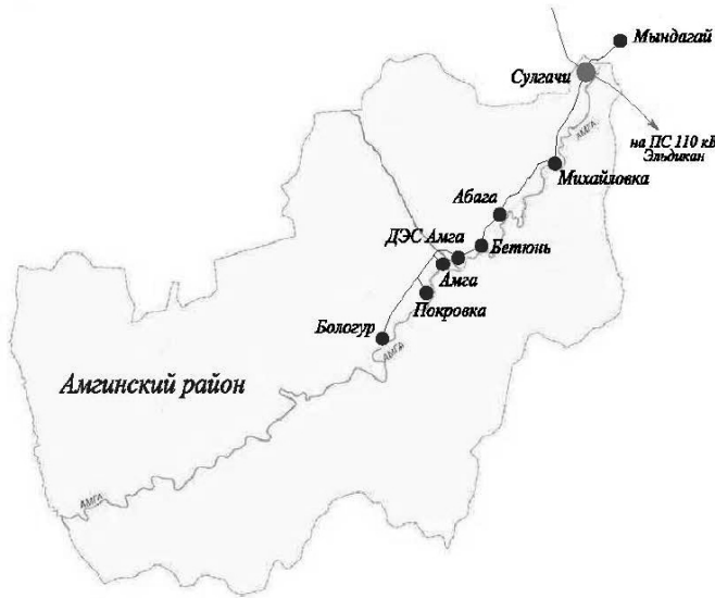
Рисунок 3.2.2.3 – Карта-схема электрических сетей Амгинского района
