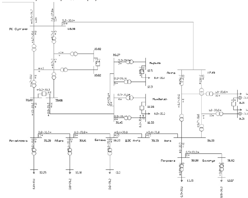
Рисунок 3.2.2.12 – Нормальный режим. Зимний максимум 2021
