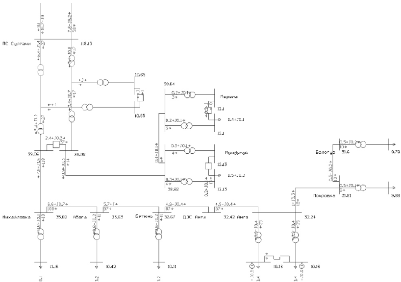
Рисунок 3.2.2.10 – Нормальный режим. Зимний максимум 2021 года
