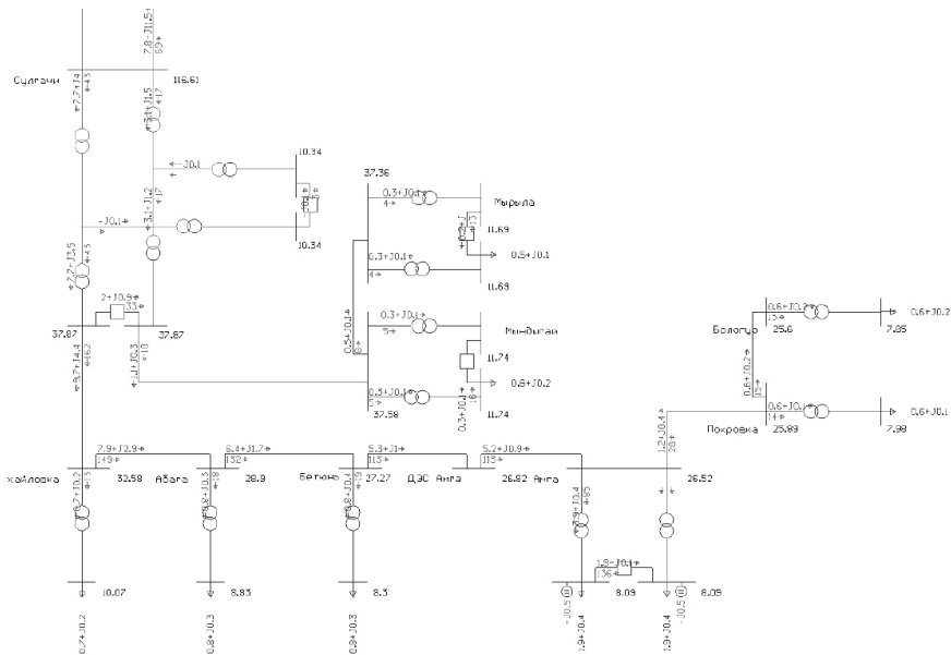
Рисунок 3.2.2.8 – Ремонт Т2 ПС 35 кВ Амга. Зимний максимум 2021 года
