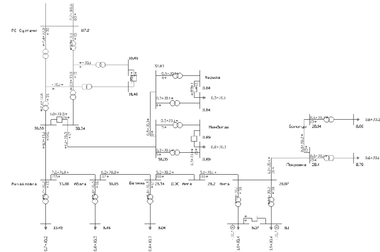
Рисунок 3.2.2.5 – Нормальный режим. Зимний максимум 2021 года
